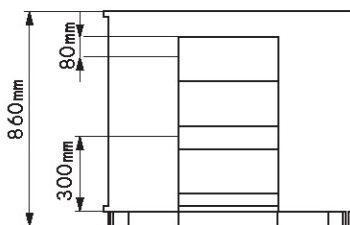
櫥櫃高度(860mm)示意圖
