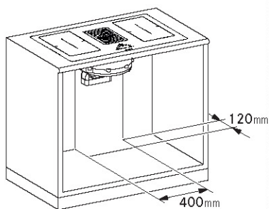
櫥櫃底板開孔尺寸
