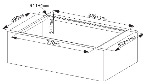
平接開孔尺寸
