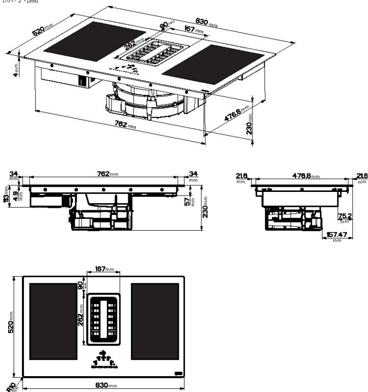
商品尺寸標示圖
